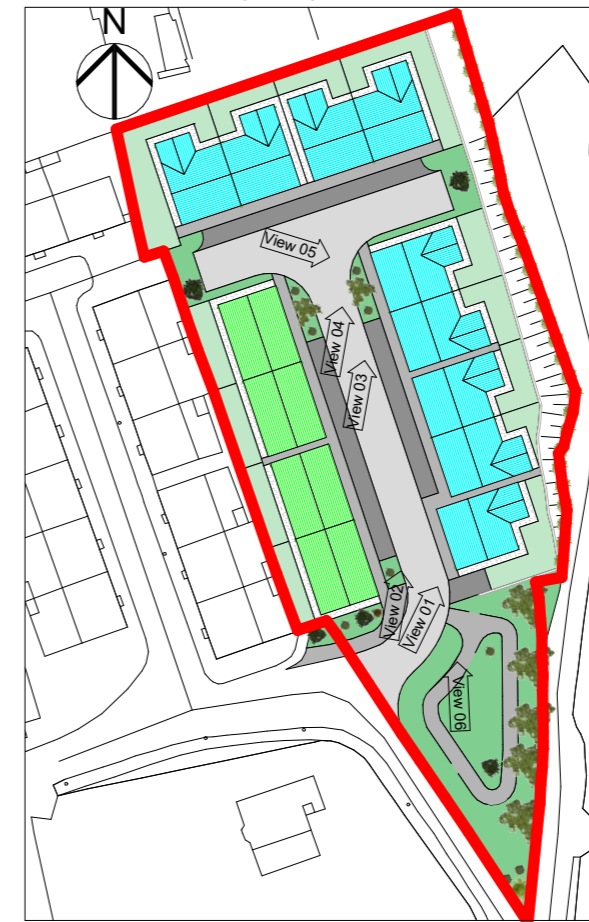
2 Site Key Plan 1:1000
